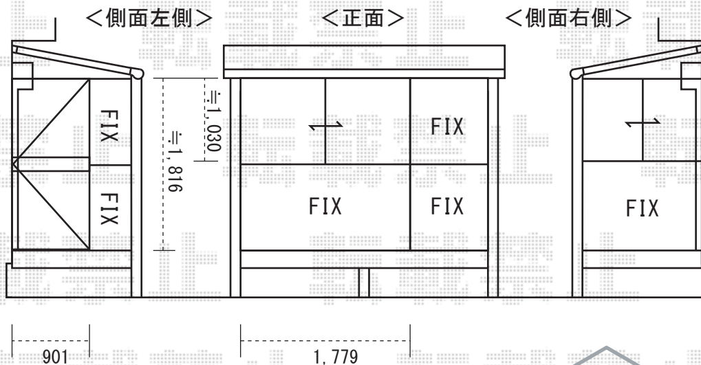
お見積2 【右側面ユニット：高窓(2枚建て) 左側面ユニット：ドア(中棧付き)】
