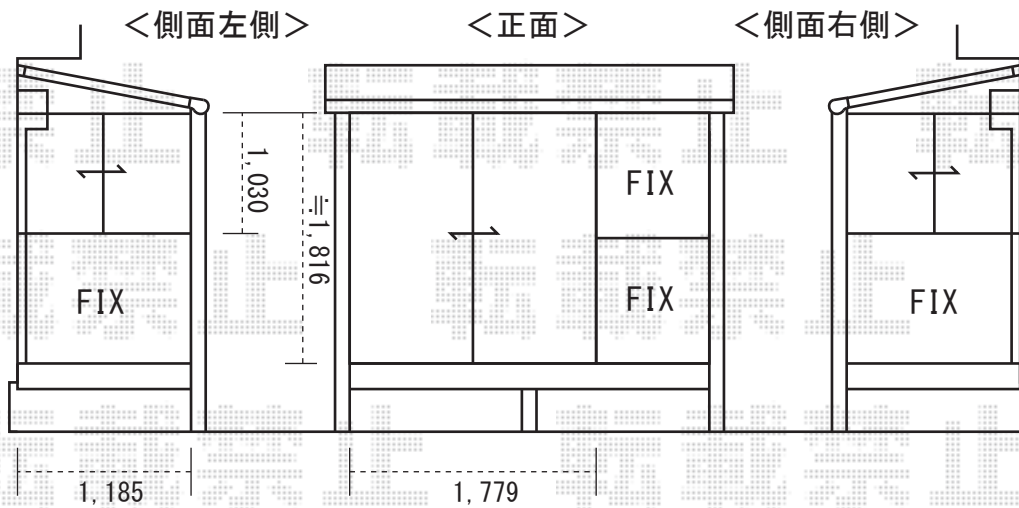
お見積1 【両側面ユニット：高窓(2枚建て)】
