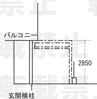
<断面図>
