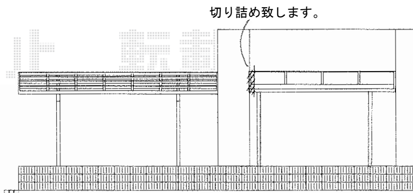
東立面図
