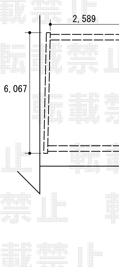
側面図
