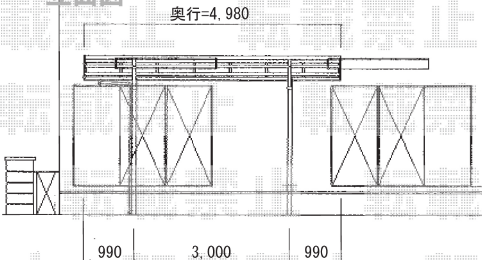
立面図
