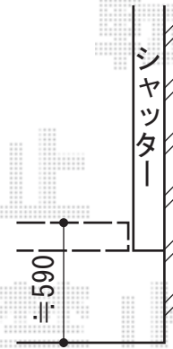
【側面納まり】
