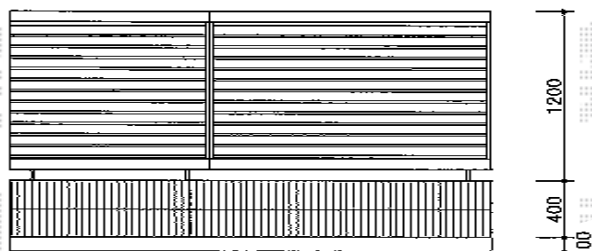
フェンス部詳細図 1/50
