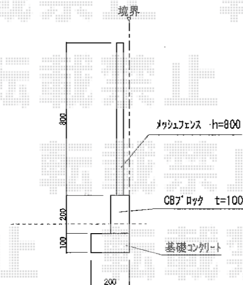
外周化粧ブロック詳細図
