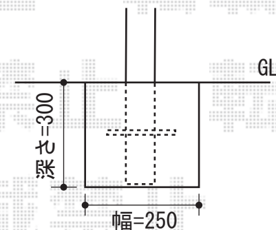
〈基礎概略図〉
