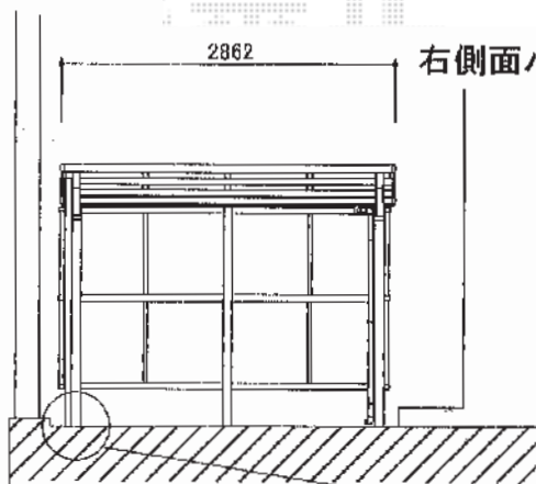
【前面図】
