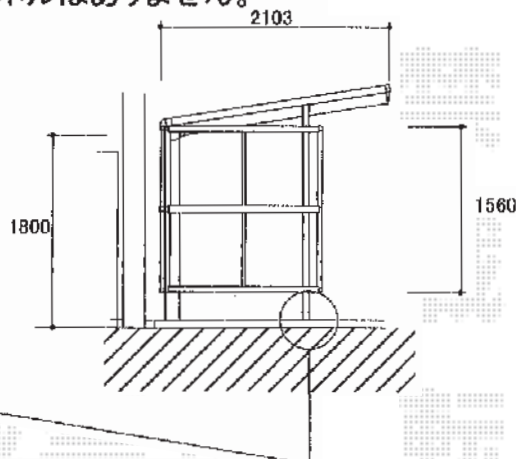
【左側面図】
