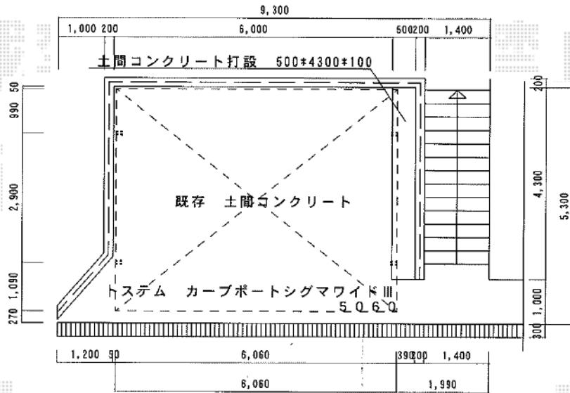
平面図 1:100
