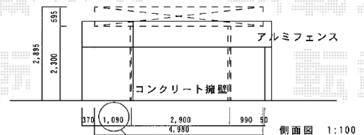
側面図 1:100
