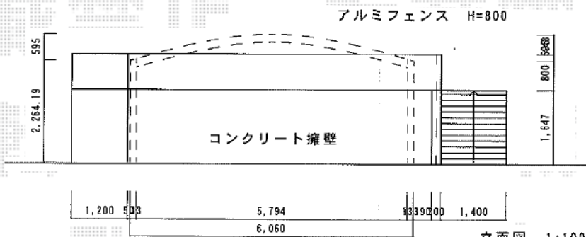
立面図 1:100
