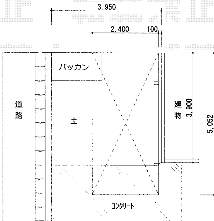
平面図
