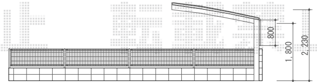
立面図 S:1/100
