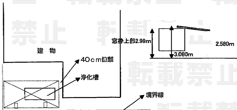
カーポート奥柱位置拡大図
