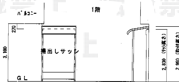
プレシオステラス (一般) 1間×4尺 物出しセット 熱線遮断ポリカーボネート
