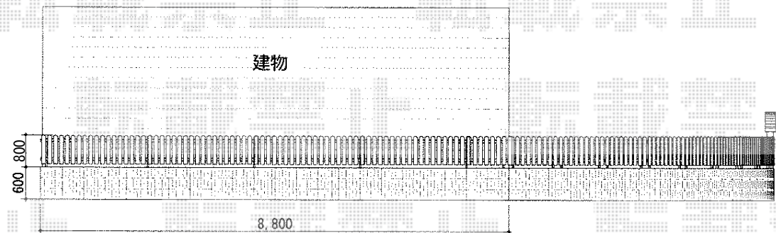
西側立面図
