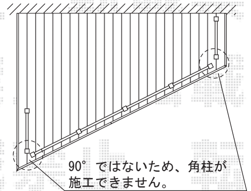
※フェンス配置図（門扉同様柱施工）
