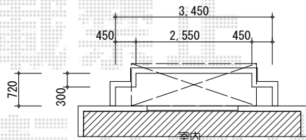
西側2Fベランダ寸法
