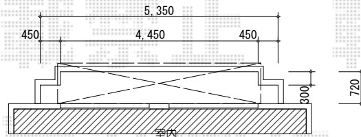
南側3Fベランダ寸法
