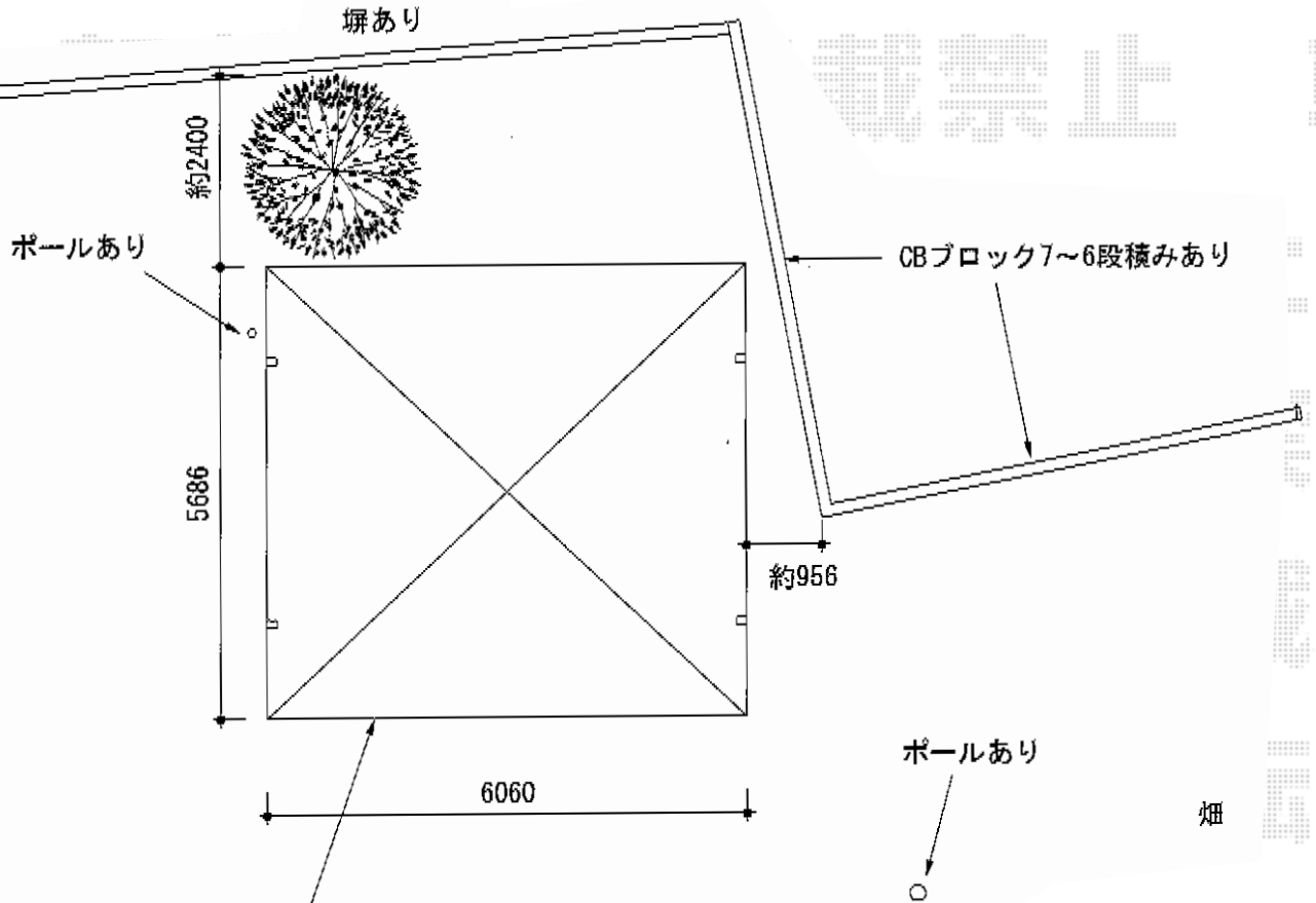
カーブポートシグマIII 5760 ロング柱23 オプション 両側サイドパネル2段(高さ=800+800) 57×2 (ロング柱23用)
