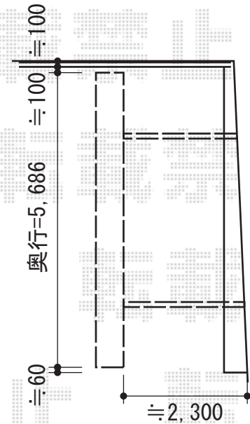
トステム カーポートシグマIII 積雪～30cm対応
