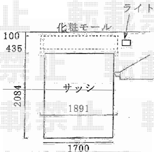
2F通路断面図
