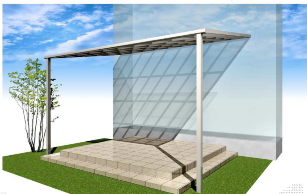
TOSTEM/パワーアルファF型/1500タイプ/メーター仕様 2間*9尺/4215*2685/標準柱
