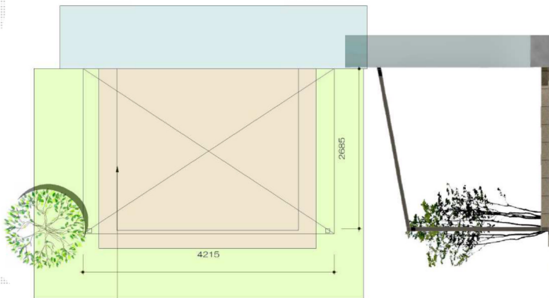
TOSTEM/パワーアルファF型/1500タイプ/メーター仕様 2間*9尺/4215*2685/標準柱
