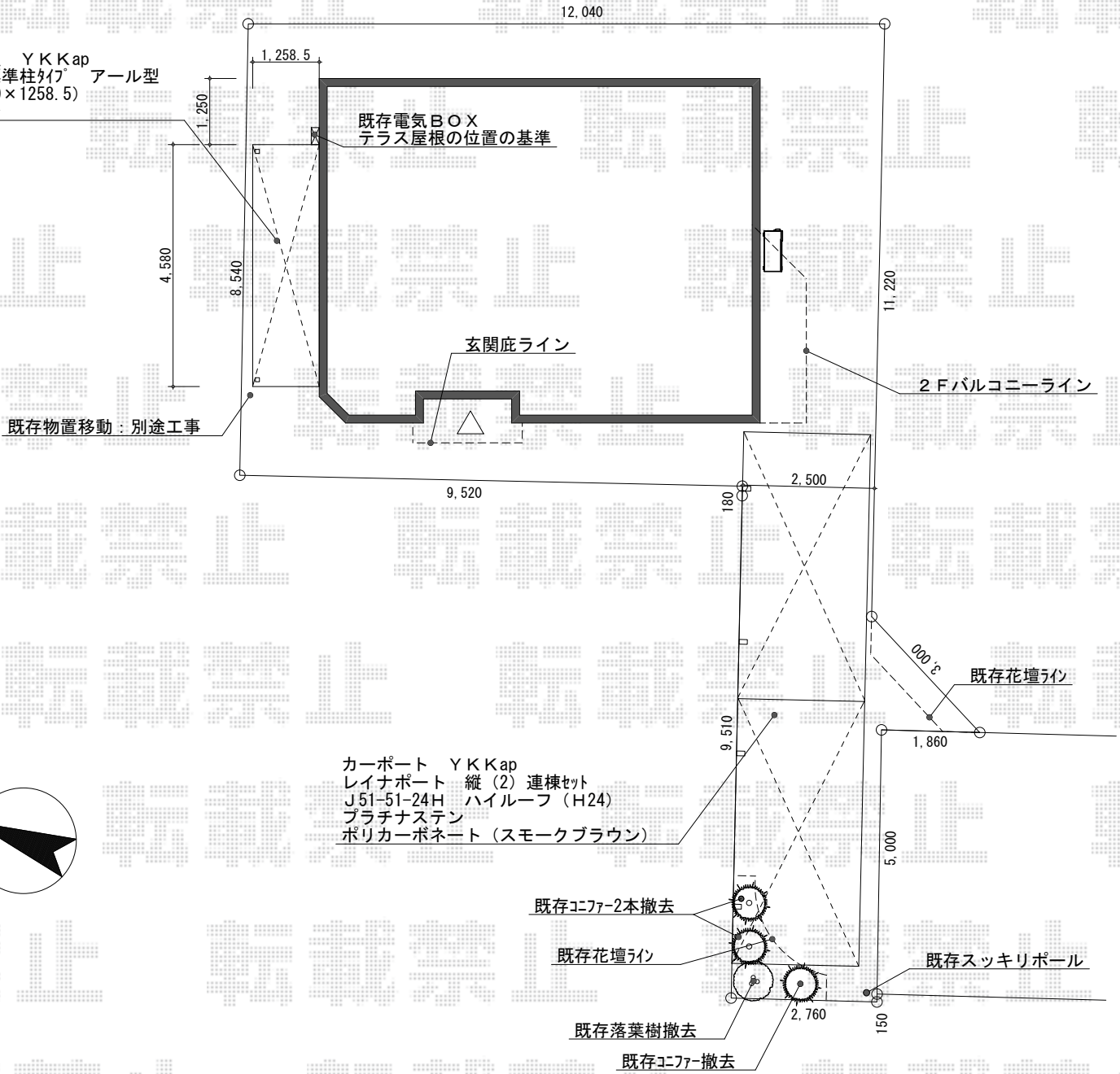
平面図 S:1/100
