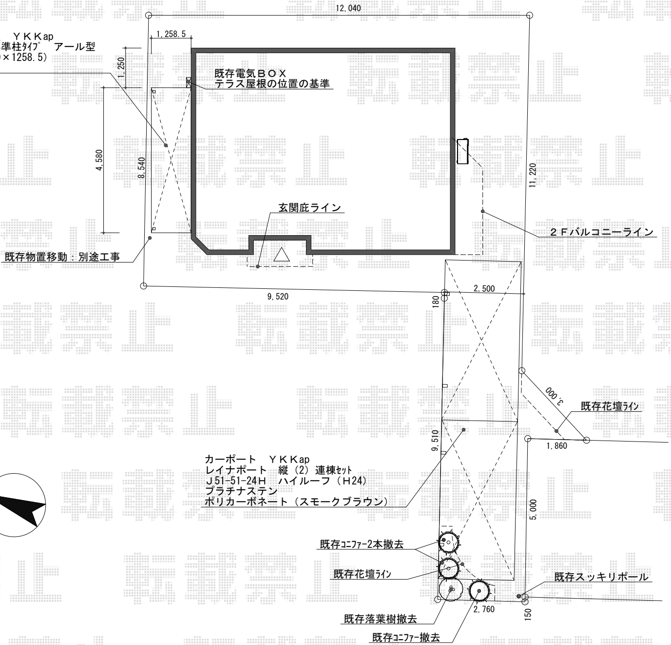
平面図 S:1/100
