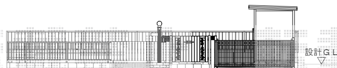
立面図
