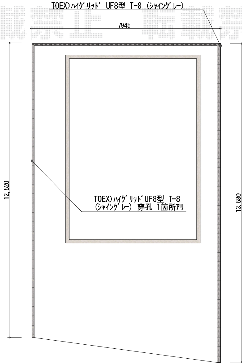
平面図
