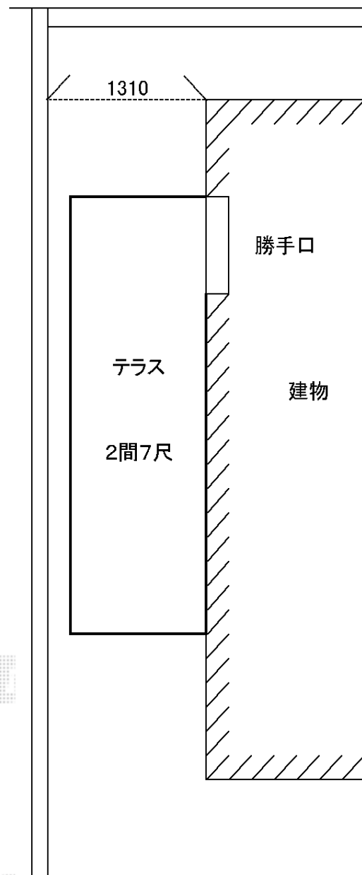
平面図
