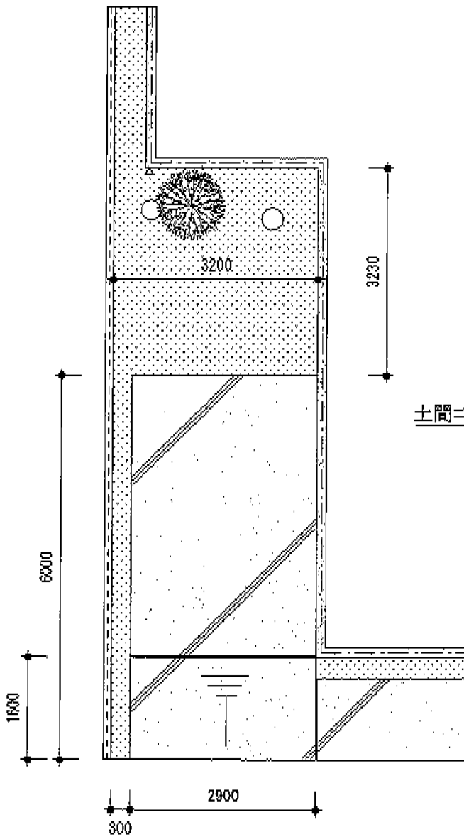
- 現況図 -
