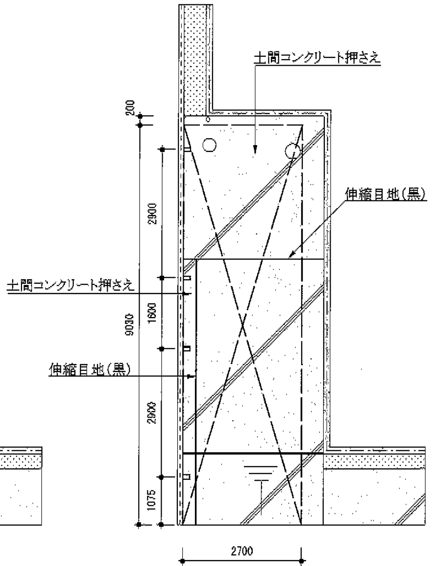
- 完成予定図 -
