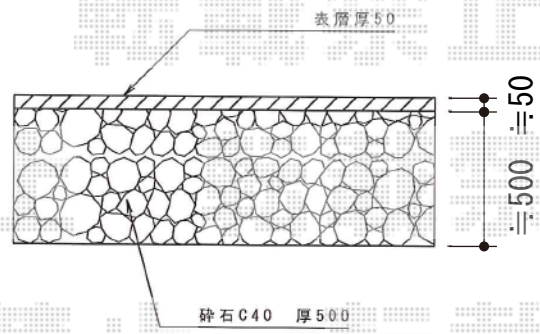
寒冷地用舗装構成
