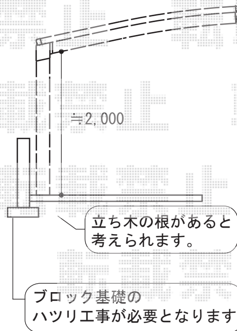
横断面図
