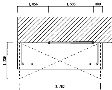
外観左側
