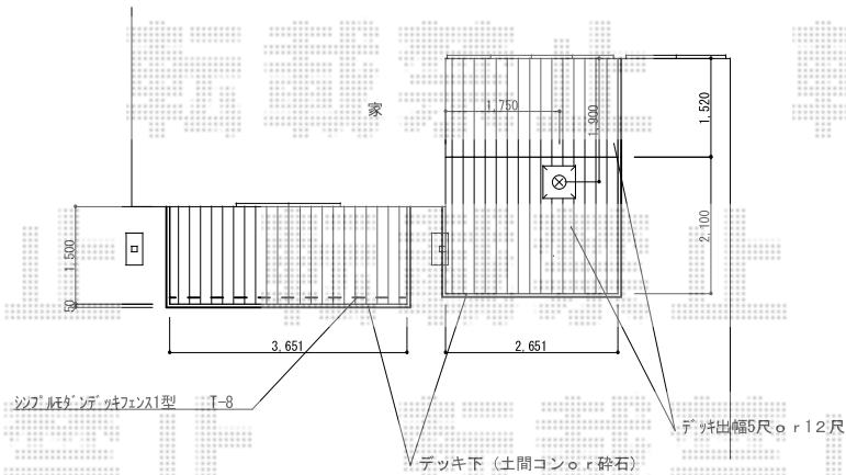
<西側：2間×7尺>
