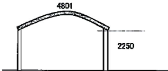
横断面図
