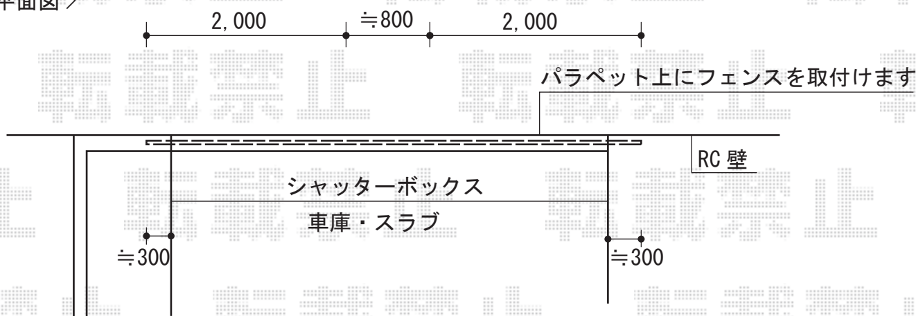
< 平面図 >
