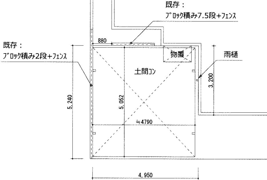
平面図 S:1/100
