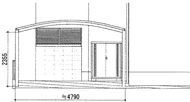
南側立面図
