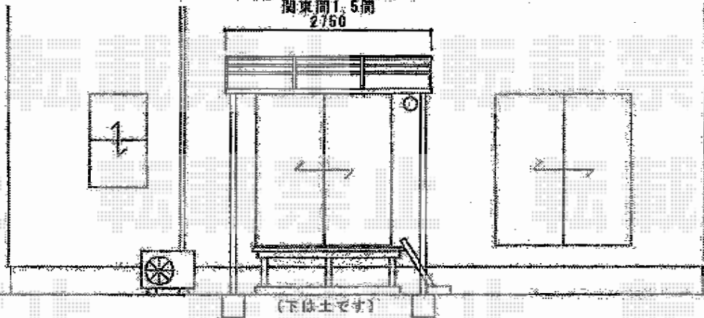
立面図
