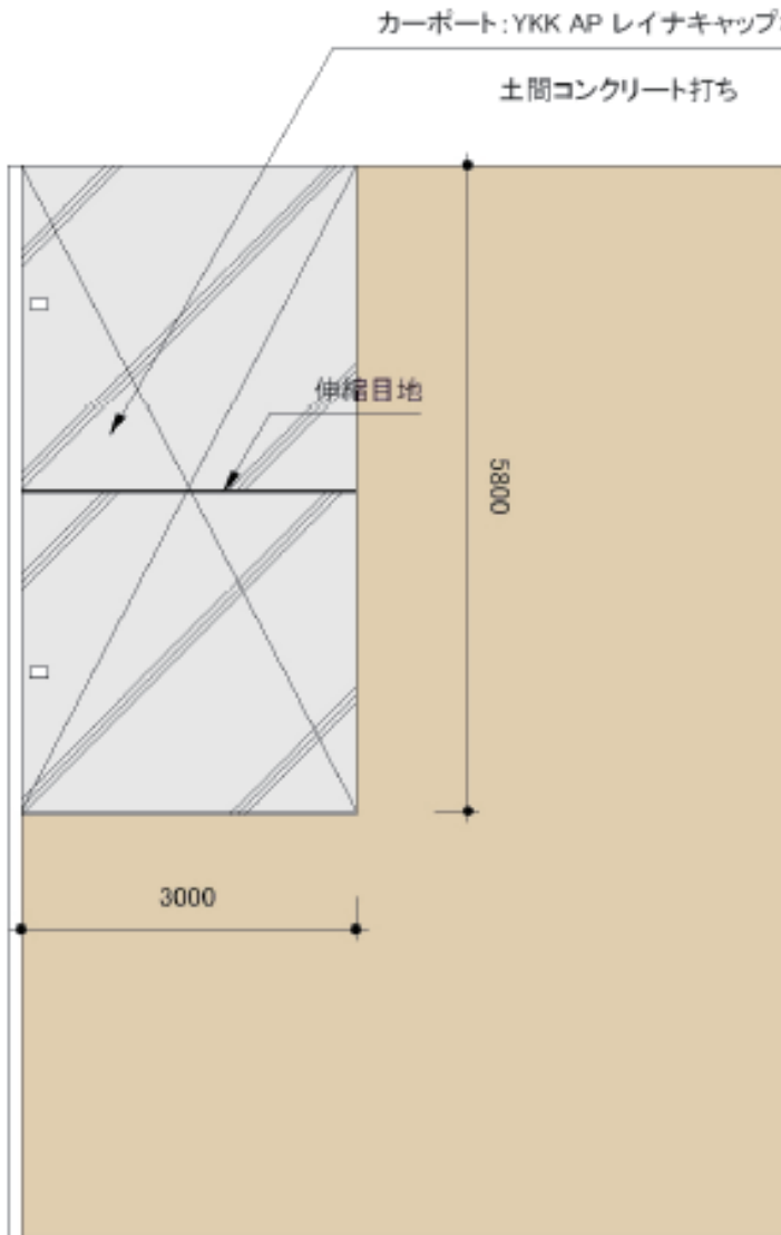
平面図 S1/100
