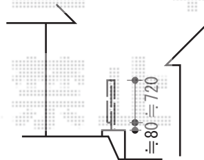
フェンス断面
