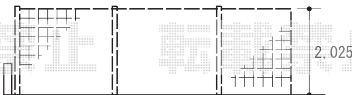
<ハイグリッドフェンス剣先1型>
