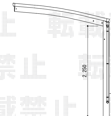
道路側柱有効高
