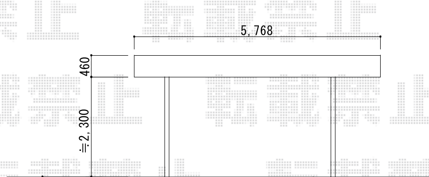
※レイナポートグラン納まり図
