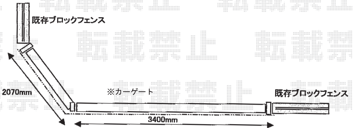
上面図
