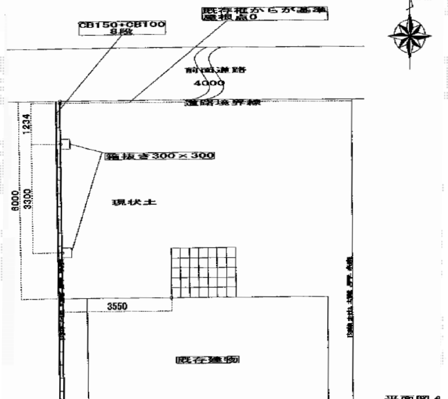
平面図A
