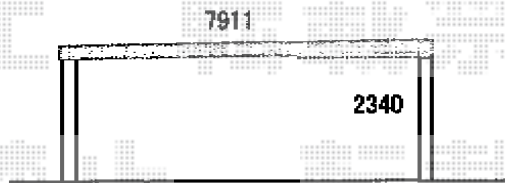
横断面図
