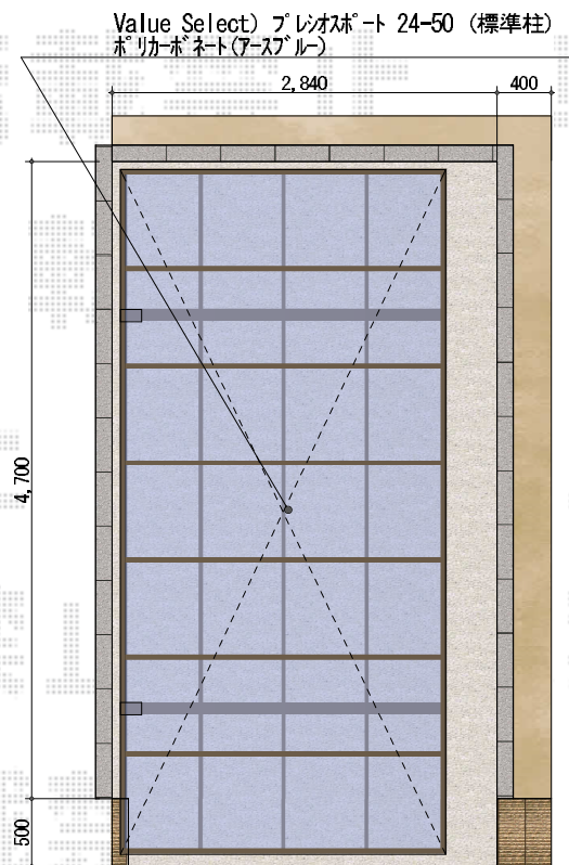
平面図
