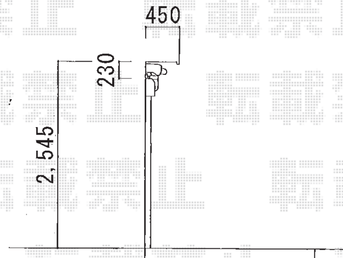
(側面図)
