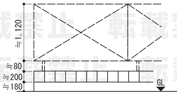
≪ブロック1段積/新設フェンス図≫
