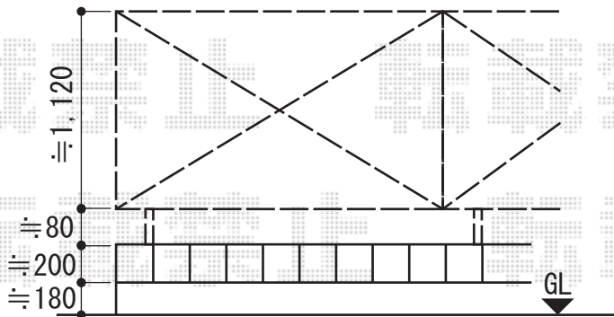
《ブロック1段積/新設フェンス図》
