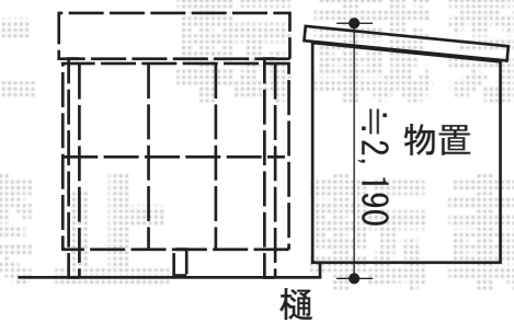
新設サイクルポート パネル1面囲い
