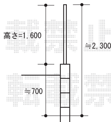
【隣地フェンス・側面図】
