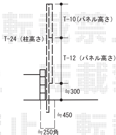
【新設フェンス・側面図】
